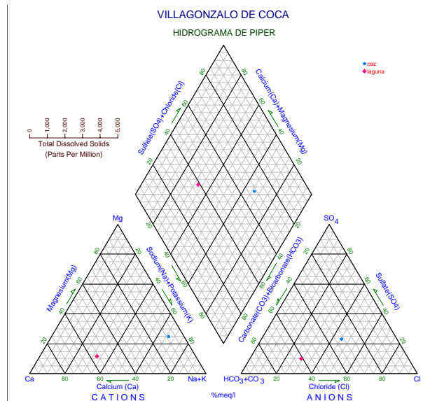
Figura 18. Hidrograma de Piper-Hill-Langelier con representación del agua de recarga artificial y la medida en el cuenco de la laguna de la Iglesia de Villagonzalo de Coca en febrero de 2006.
